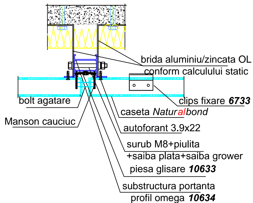
Sectiune orizontala
